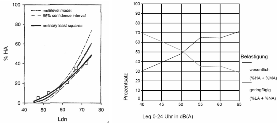
Figur 4 Dosis-Wirkungskurven (%HA als Funktion des Ldn bzw. Leq 0-24) für Fluglärm. Aus Miedema & Vos (1998) und Wirth (2004).
