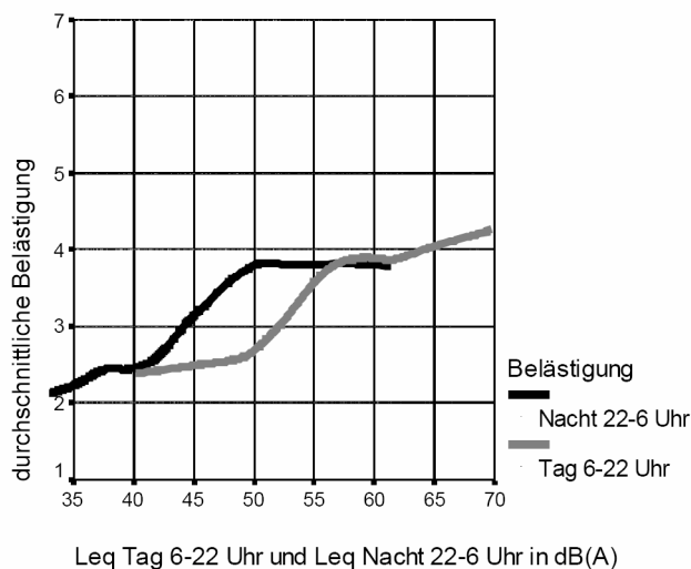
Figur 5 Fluglärmelastigung (1 = überhaupt nicht belästigt, 7 = unerträglich belästigt) nachts aufgrund des Leq 22-6 Uhr und Fluglärmelastigung tagsüber aufgrund des Leq 6-22 Uhr. Kurve eingepasst nach der Lowess-Methode. Stichprobe mit Zivilfluglärm, N=1215. (Quelle: Wirth 2004).
